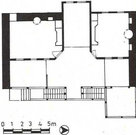
Çizim 4— Bozerler Evi üst kat planı
