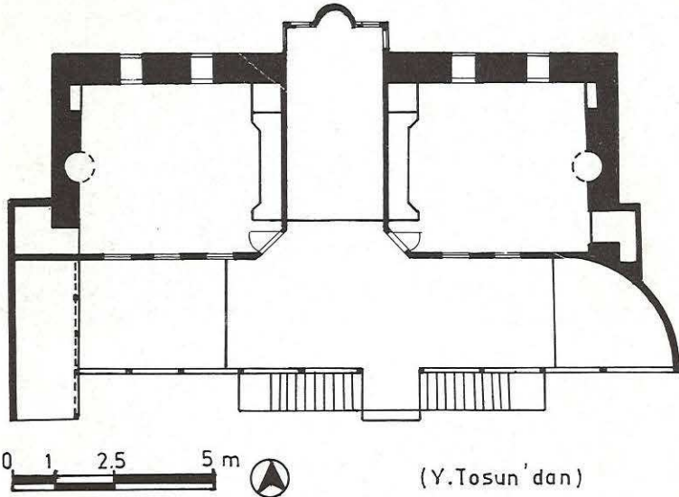
Çizim 3 — Hacı Recepler Evi üst kat planı
