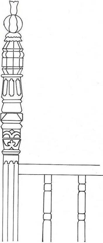
Çizim 20 — Merdiven babası (Beyoğlu Evi'nden)
