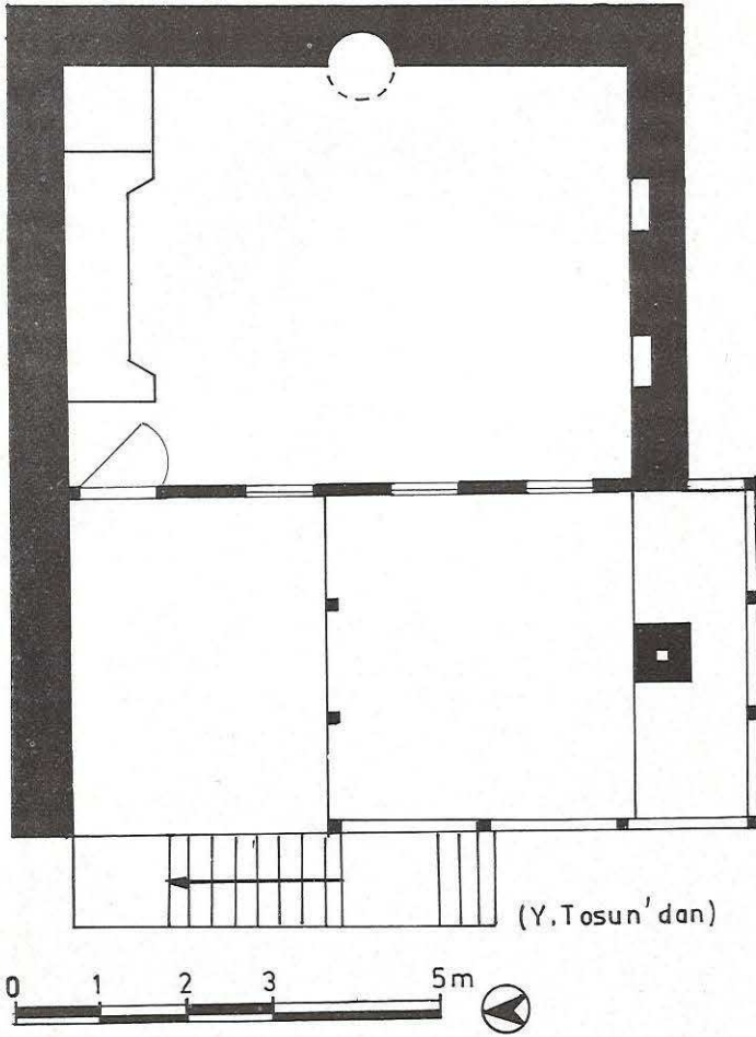
Çizim 7 -- Kızıklar Evi üst kat planı
