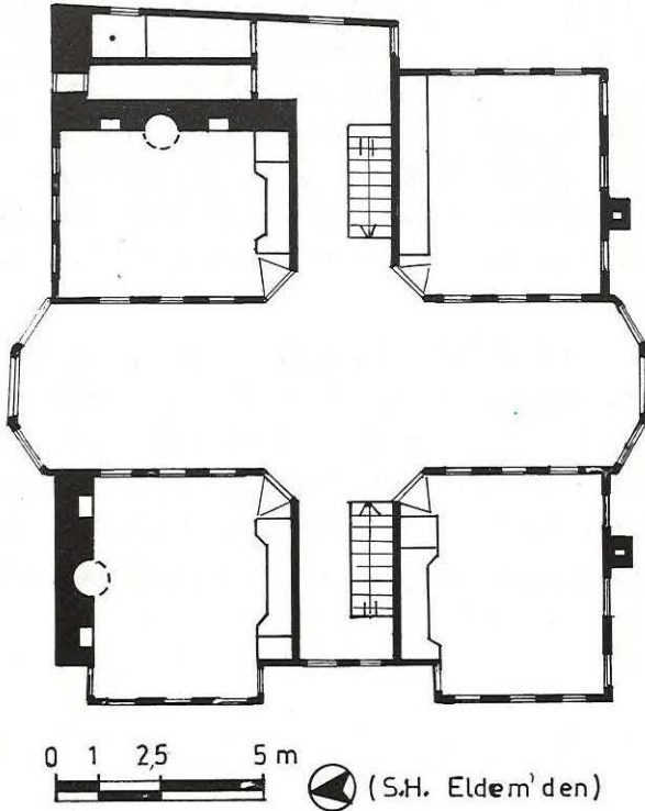
Çizim 5— Küçük Göldeliler Evi üst kat planı
