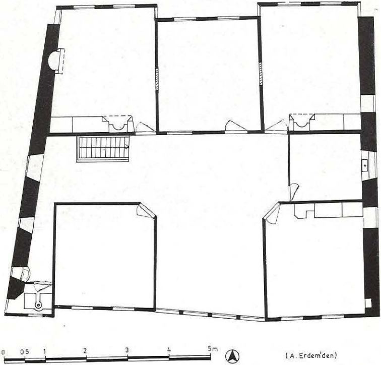
Çizim 6— Beyazoğlu Evi üst kat planı
